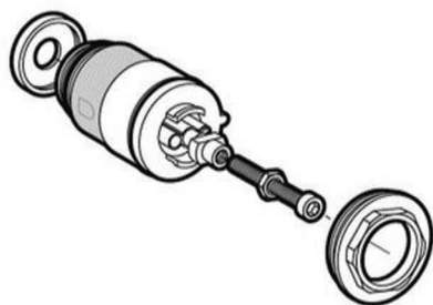
Μηχανισμός για Εντ/νο Φλουσόμετρο WC Edition #296260099
